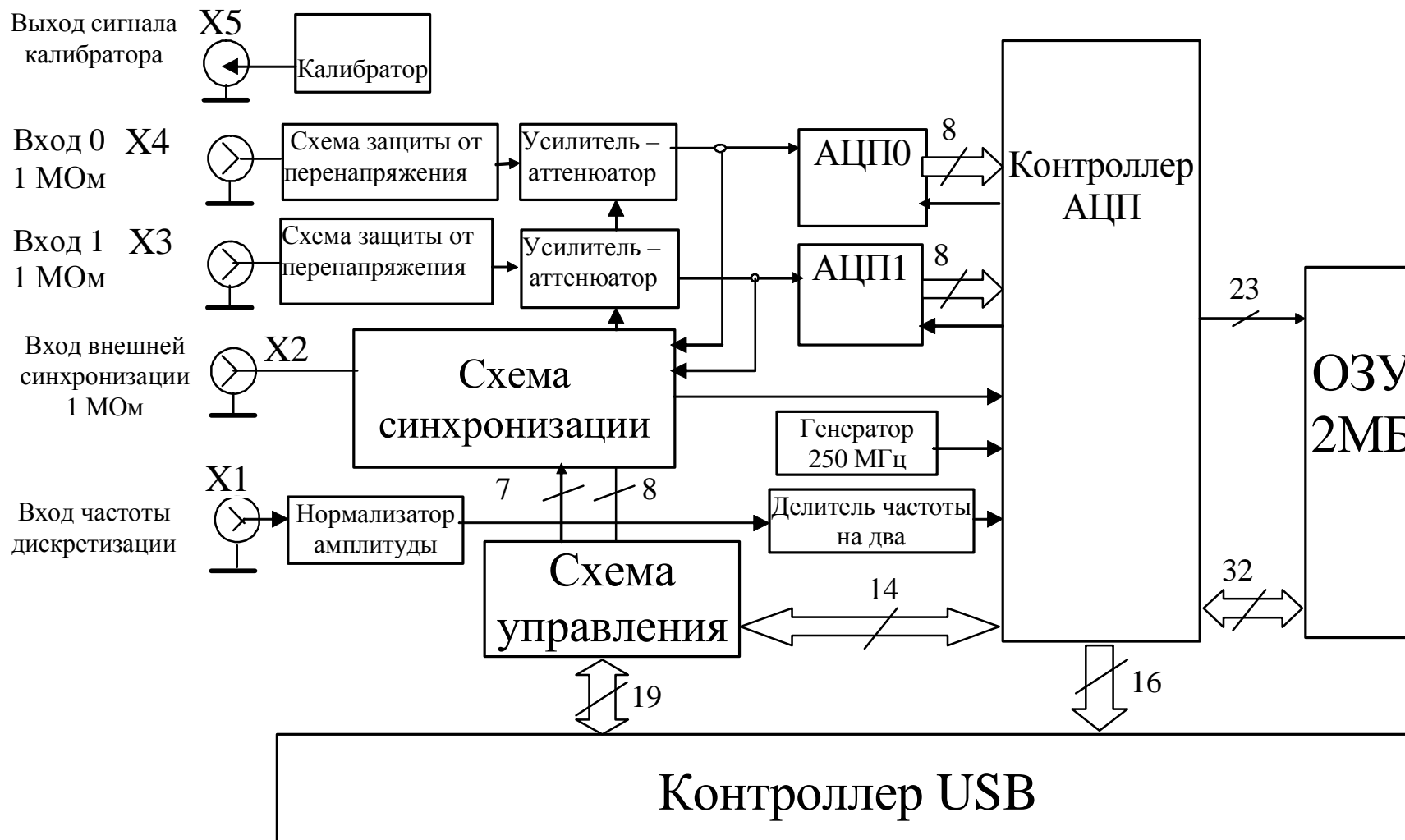
Рис. 5.1 Функциональная схема ОЦЗС-02(250USB)
